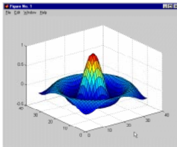
Figura 16. Función "sombbrero" con facetas.
