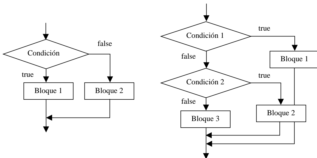
Figura 17. Ejemplos gráficos de bifurcaciones.
