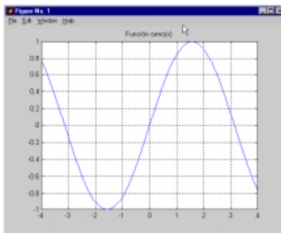
Figura 2. Gráfico de la función \text{seno}(x) .
