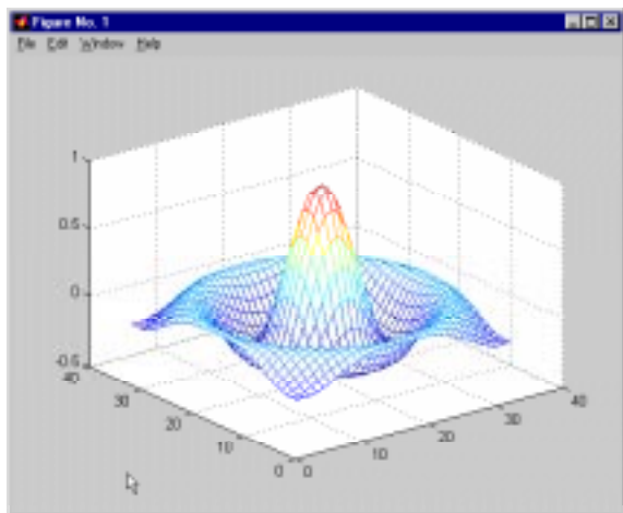
Figura 15. Figura 3D de la función "sombbrero".
